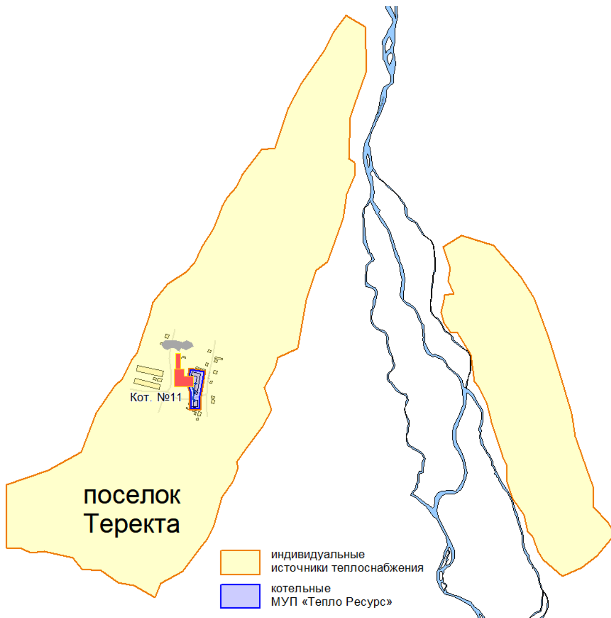
Рисунок 3.1 – Зона действия источников тепловой энергии п. Теректа
