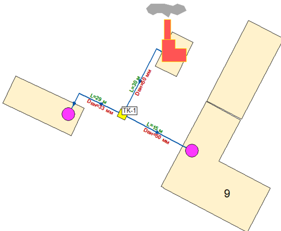
Рисунок 2.6 – Схема тепловых сетей в зоне действия котельной №17, с. Абай
