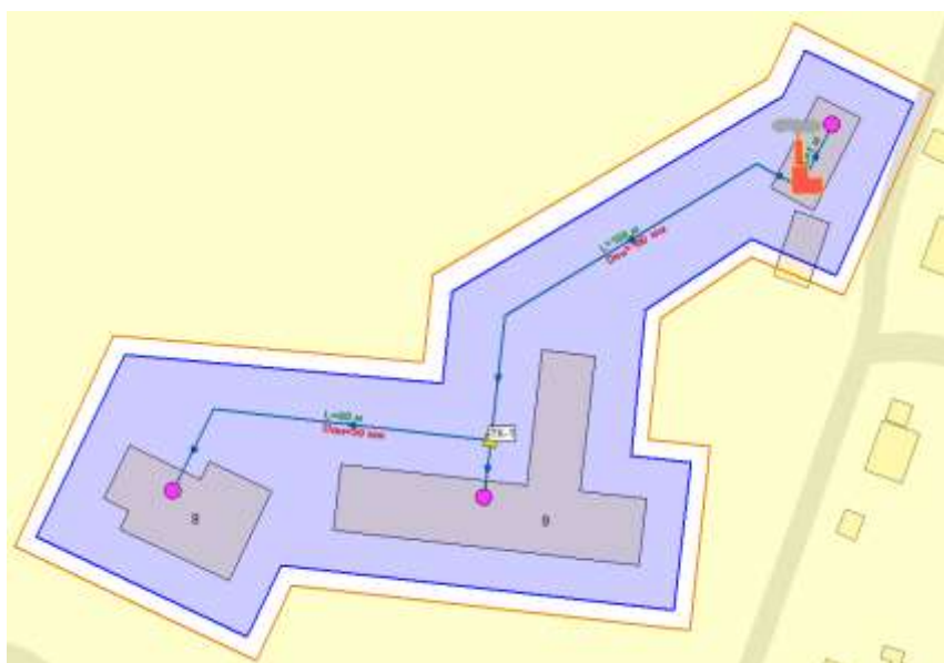
Рисунок 4.6 – Зона действия котельной №16 (с. Амур)
