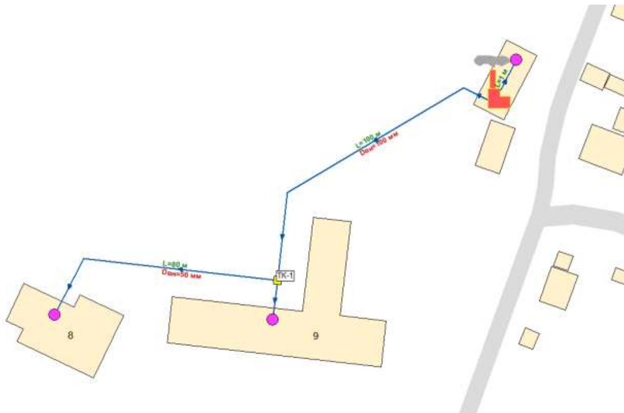
Рисунок 2.5 – Схема тепловых сетей в зоне действия котельной №16, с. Амур
